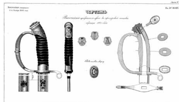
Чертёж эфеса офицерской драгунской шашки образца 1909 года с расположением на нём и клинке герба и вензелей [9].
