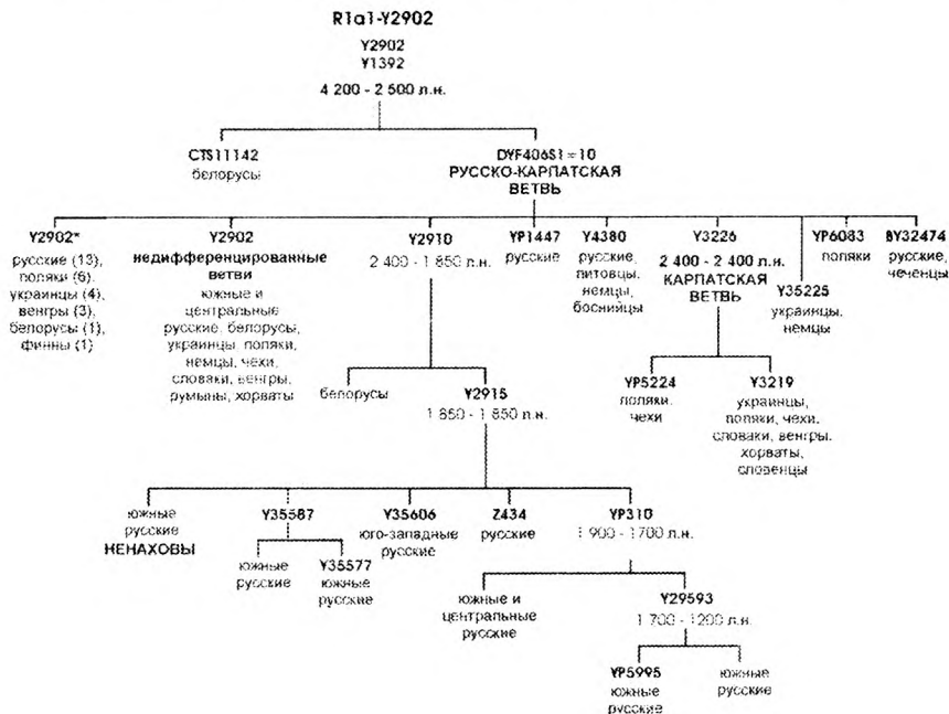
Рис. 1. Филогенетическое древо линии R1a1-Y2902 .
