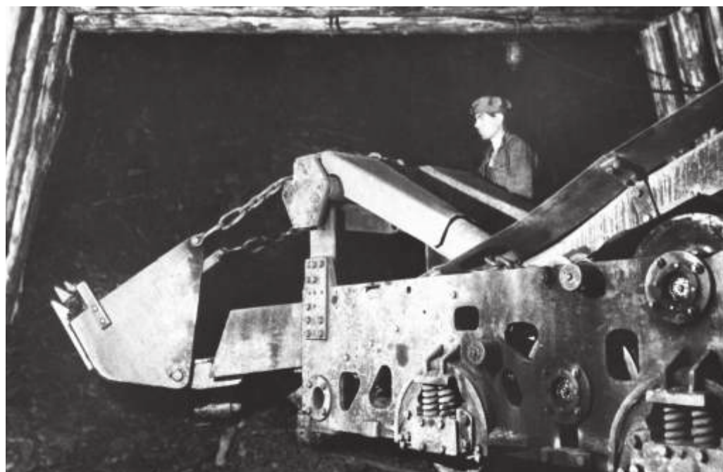
В забое шахты 3-ц треста «Артемуголь». Приморский край, г. Артем. 1953 г. Автор: Ткаченко М.Г. // ПГОМ. МПК 2369—8. Ф 12951
